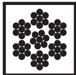
Drahtseil 6x7 mit Stahleinlage
