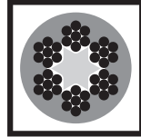
Drahtseil 6x7 Kunststoffummantelt
