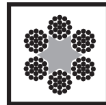
Câble métallique 6x19
