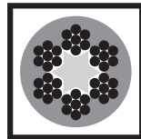
Câble métallique 6x7, gaine en plastique
