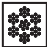
Drahtseil 6x7 mit Stahleinlage
